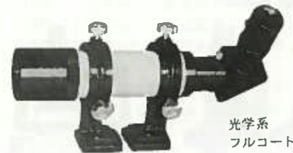
• 11X40mmファインダーDP 天頂プリズム付(反射式用) 取外し可能 対物レンズ:アクロマート D40mm F220mm 接眼レンズ:K20mm十字線入(24.5mmサイズ取外し可能) 総重量400g 長さ21cm 二本脚付7,000円・脚なし5,500円
