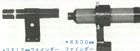
• 3X12mmファインダー 小型軽量 重量45g 長さ91mm 十字線入 1,400円 • 6X30mmファインダー 重量150g 長さ145mm 一本足付 十字線入 2,600円
